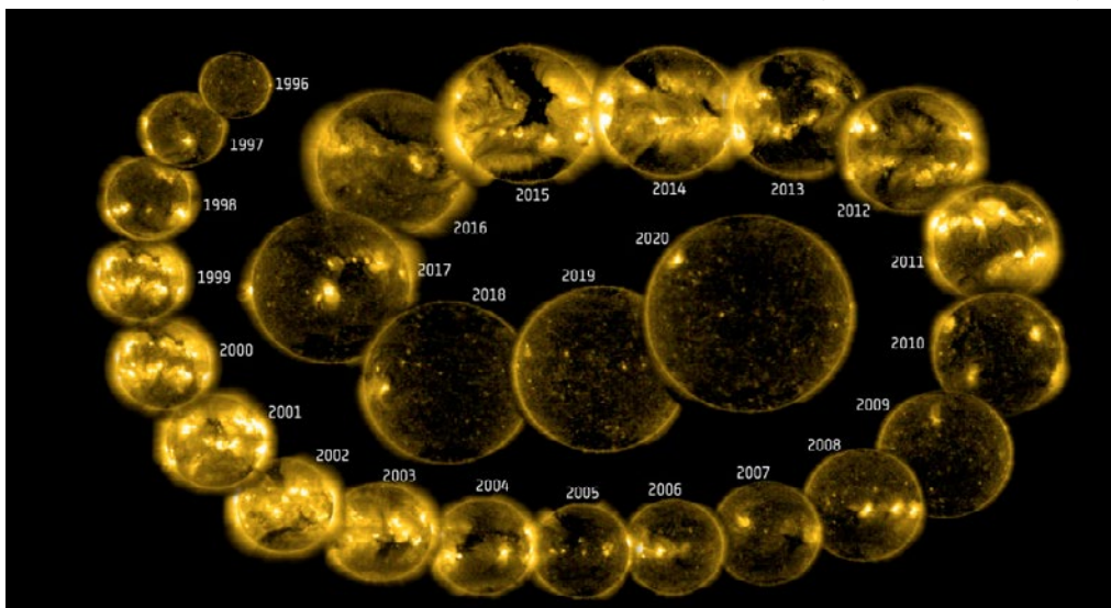
Aktivita Slunce 1996–2020
